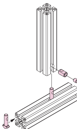
KFジョイントキット4045H (フレームに対して、側面から固定します)
