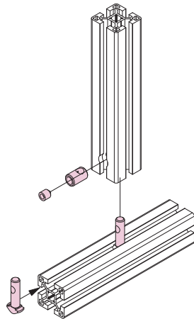
KFジョイントキット4045V (フレームに対して、正面から固定します)
