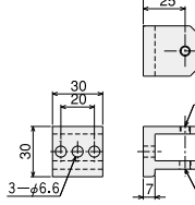
ターンブラケット30A レバータイプ
