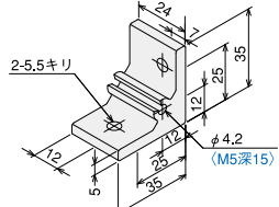
ハードブラケットS-SS-R
