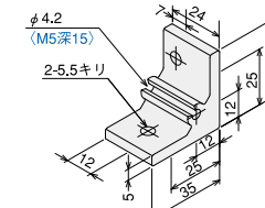
ハードブラケットS-SS-L
