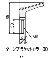
クランプレバー-30
