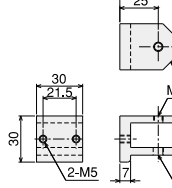
ターンブラケット30B レバータイプ
