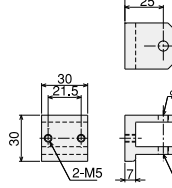
ターンブラケット30C レバータイプ
