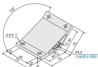
ハードブラケットL4590・DE135
