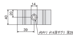
トラスジョイントL40
