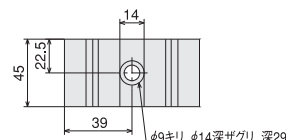
トラスジョイントL45
