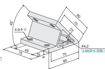
ハードブラケットL4590・DE45
