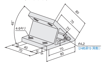
ハードブラケットL4080・DE45
