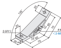
ハードブラケットL・DE135
