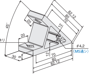
ハードブラケットL・DE45
