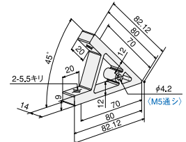
ハードブラケットSS・DE45
