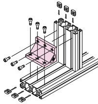
ハードブラケットS3090
