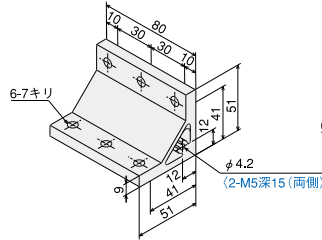
ハードブラケットS3090
