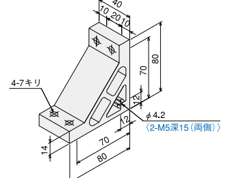
ハードブラケットSG50
