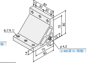
ハードブラケットSG3090
