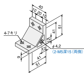
ハードブラケットS50
