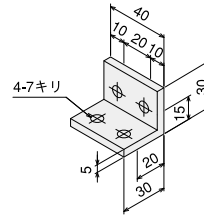
アングルブラケットS50
