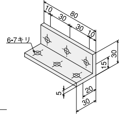
アングルブラケットS3090
