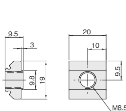
アルミナットL(M8.5)
