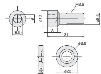
アルミボルトM8.5×23/アルミワッシャー(M8.5)
