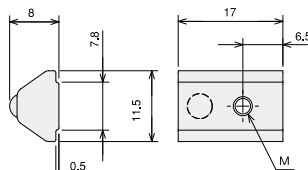
EasyナットS B
