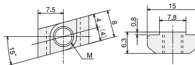
SフリーナットS B
