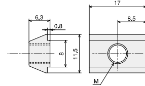
アフターナットS B
