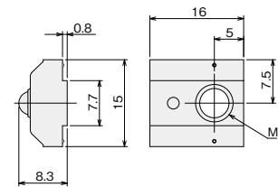
STナットストッパー付きS B
