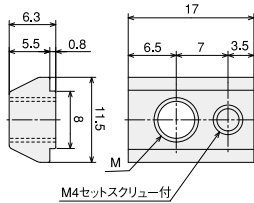
後入れロックナットS B
