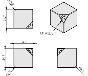
3方ブロック 40キャップ (ステンレス)
