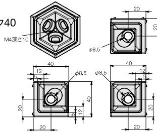
3方ブロック 40キャップ
