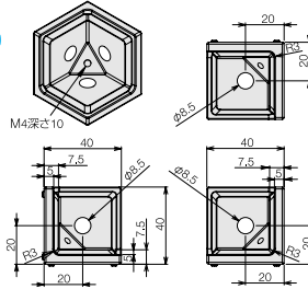
3方ブロック40 (ステンレス)
